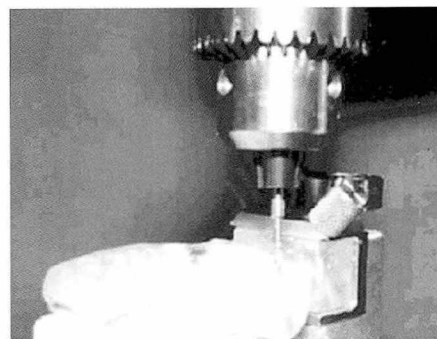
그림 3. 드릴을 이용한 스텐트에 가이드 홀 제작
