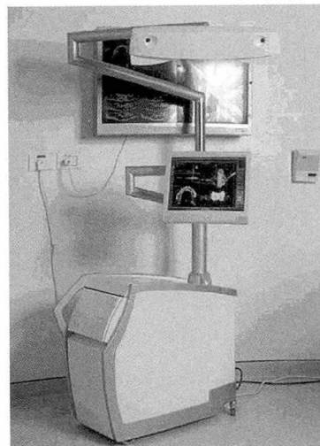
그림5. 광학적 위치추적을 이용한 영상유도 임플란트 시술 시스템의 한 예, DenX:Israel
